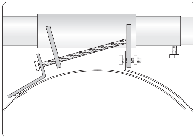
Spændebånd monteres på beslag. Det er vigtigt at båndet monteres på den indvendige side af beslaget. Beslaget monteres på teleskopstang.
