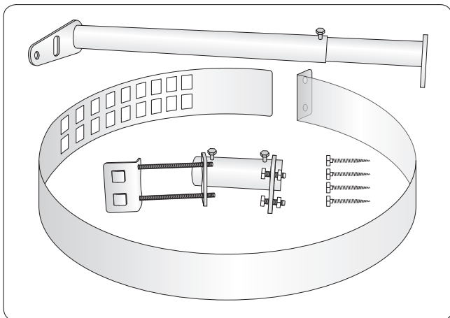
Teleskopstang - Beslag - Spændebånd - 4 Træskruer
