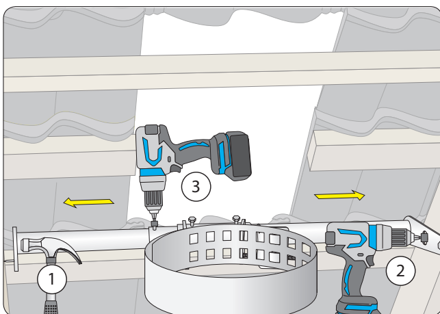
Teleskoprør monteres på spær (afstand fra 700 til 1250 mm)
