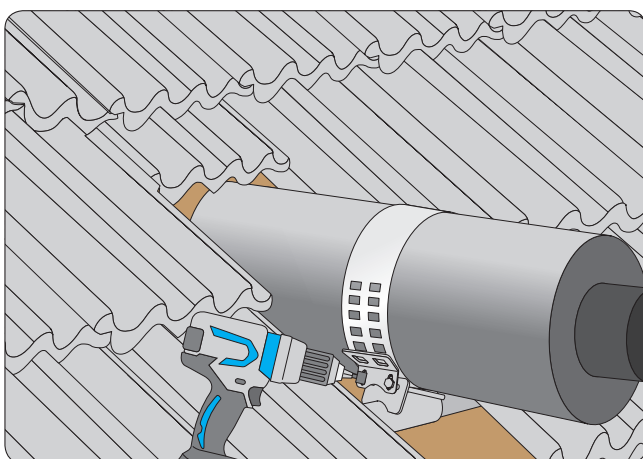
Spænd de to lange skruer ind, til båndet er stramt.
