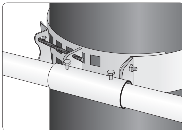
Rør føres gennem bæring og justeres i højde.
