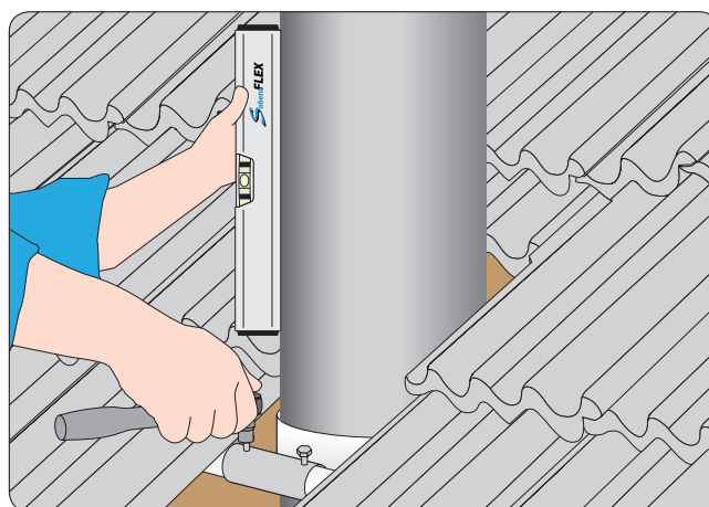
Røret rejses til lodret, og de to skruer spændes.
